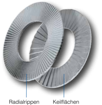
Radialrippen Keilflächen
